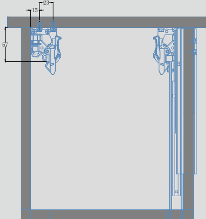
把手安装图 (b) Handle Ins. b
