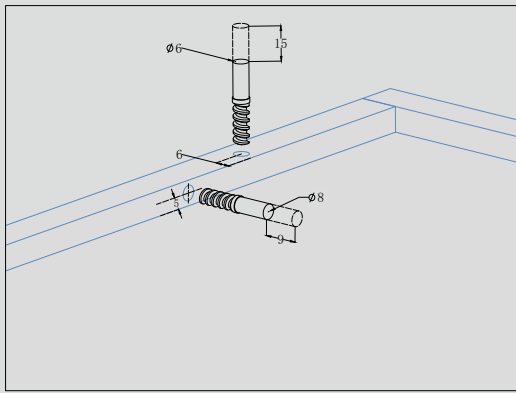
抽屉侧板-打孔直径及深度 Drilling Distance
