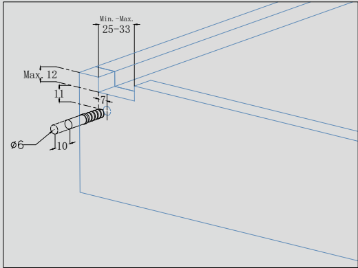
8 把手安装图 (b) Handle Ins. b
