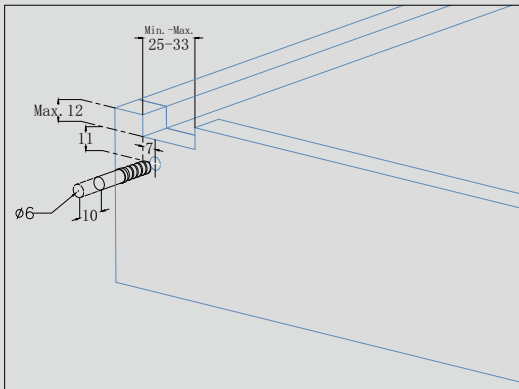
7 抽屉背板-打孔直径及深度 Drilling Distance
