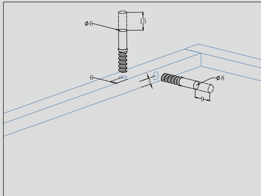
8 抽屉侧板-打孔直径及深度 Drilling Distance
