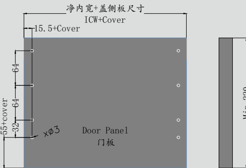
门板尺寸 Door Size
