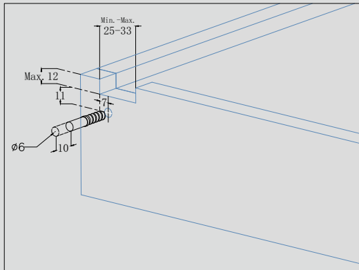
7 把手安装图 (a) Handle Ins. a
