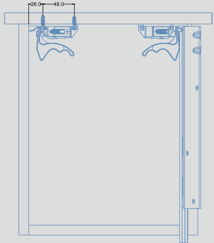
8 把手安装图 (b) Handle Ins. b
