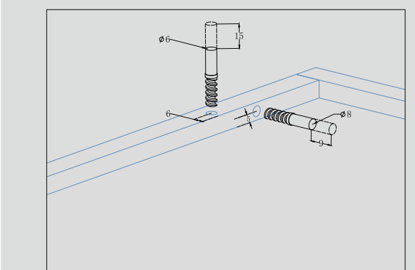
抽屜側板-打孔直徑及深度 Drilling Distance
