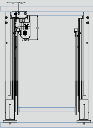
把手安装图 (b) Handle Ins. b
