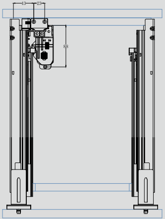
8 把手安装图 (b) Handle Ins. b
