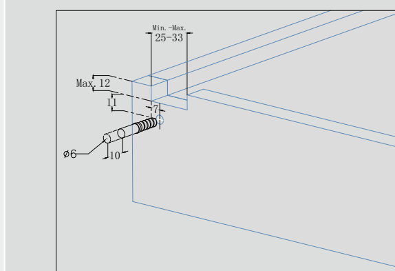
抽屜背板-打孔直徑及深度 Drilling Distance
