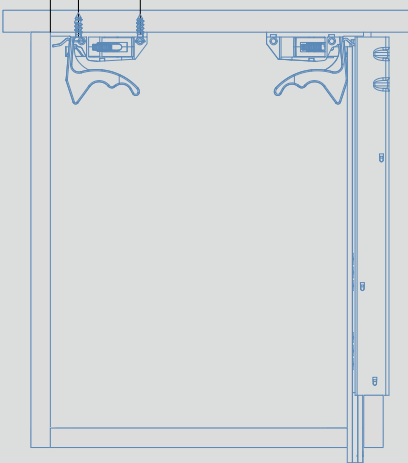
8 把手安装图 (b) Handle Ins. b
