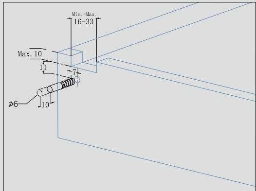
抽屉背板-打孔直径及深度 Drilling Distance
