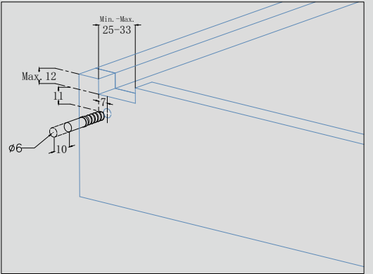
8 把手安装图 (b) Handle Ins. b
