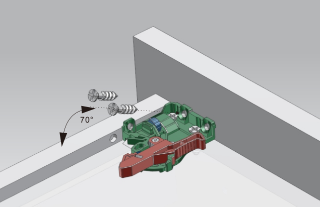
把手安装图 (a) Handle Ins. a
