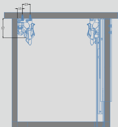
8 把手安装图 (b) Handle Ins. b
