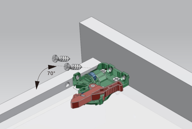
7 把手安装图 (a) Handle Ins. a
